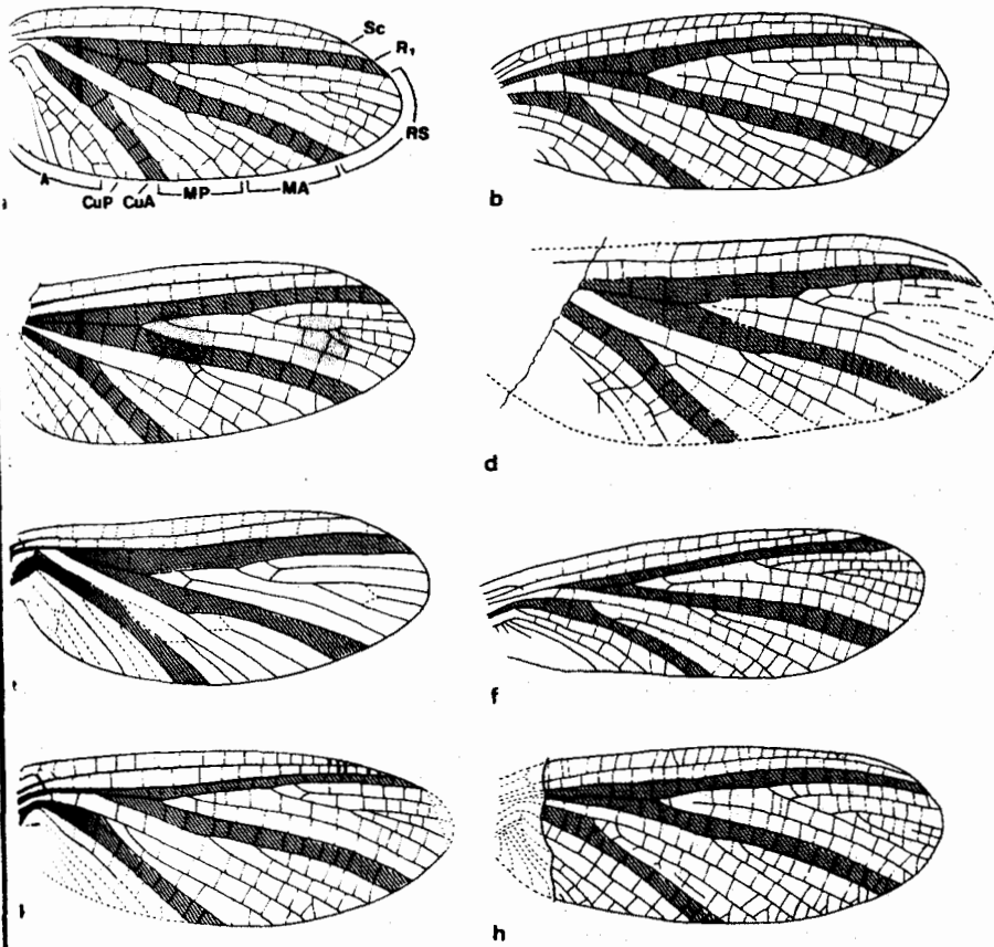
Abb. 1. Die Flügel der bisher beschriebenen Arten der Gattung Misthodotes . a) M. edmundsi (b) M. sharovi c) M. biguttatus (d) M. stapfi n. sp. e) M. delicatulus (f) M. obtusus g) M. ovalis (h) M. zelesskyi
