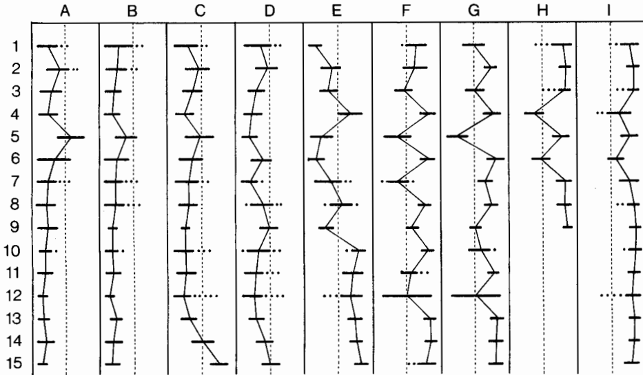
Abb. 3. Merkmalsprofile für verschiedene Populationen der pseudorivulorum -Gruppe. — A. C. beskidensis (Beskiden), — B. C. beskidensis (Wieslauf, Baden-Württemberg), C. C. beskidensis (Lein, Baden-Württemberg), — D. C. beskidensis (Fulda), — E. C. (?) pseudorivulorum (Holland), — F. C. pseudorivulorum belfiorei ssp. n. (Kalamas-Fluß, Griechenland), — G. C. pseudorivulorum belfiorei ssp. n. (Fiume Solinello, Italien), — H. C. pseudorivulorum (Main), — I. C. pseudorivulorum (Warta).
